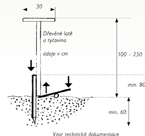
Vzor technické dokumentace
